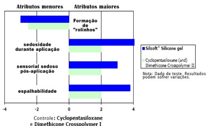
Gráfico 1: Comparação de propriedades sensoriais entre SILSOFT SILICONE GEL e elastômero de mercado.
